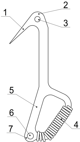
Рис. 1. 1 – клиновидное лезвие; 2 – упор; 3 – отверстие для подвешивания на рюкзак или пояс; 4 – рукоятка; 5 – перемычка; 6 – отверстие для закрепления петли для ног или оттяжки; 7 - упор.
